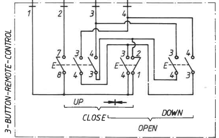
ELECTRICAL WIRING DIAGRAM LM-500/1, -750/1, -1000/1, -1500/1
